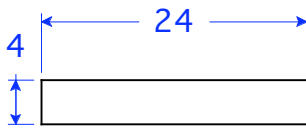
PV 4"W x 24"L x 1.5"H
