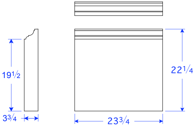
BM 26-19.5 STR 22 1/4"H x 23 3/4"L x 3 3/4"T
