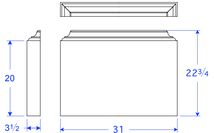
BM 26-20 DR 22 3/4"H x 31"L x 3 1/2"T
