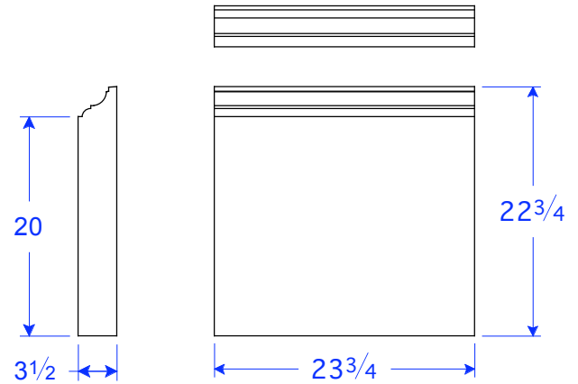
BM 26-20 STR 22 3/4"H x 23 3/4"L x 3 1/2"T
