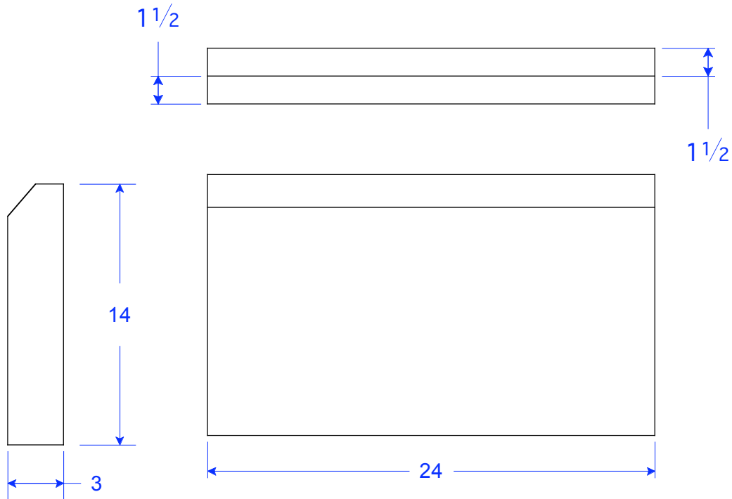
BM 34-3x14 STR 14"H x 24"L x 3"T
