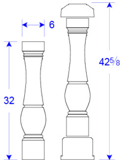
BL 01-32 BL 01-32 Set Up Weighs +/- 181 lbs per lineal foot.
