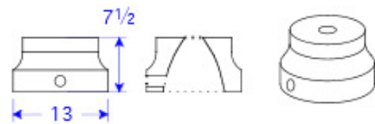
LB 01-33 Optional Base 13"O.D. x 7 1/2"H
