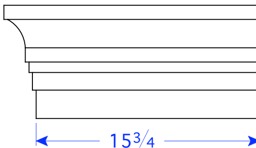
CM 8 RR 8"H x 18"L x 4 1/2"T
