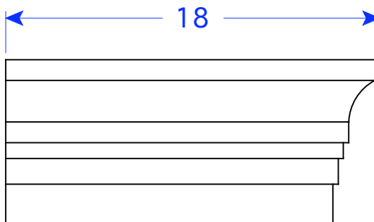
CM 8 LR 8"H x 18"L x 4 1/2"T
