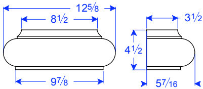
PL 01-8.5 x 4.5 DBN
