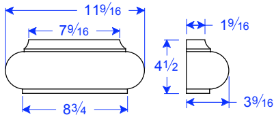
PL 01-7.56 x 4.5 DBN
