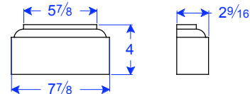
PL 18-5.75 x 4
