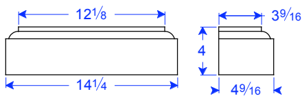
PL 18-12 x 4
