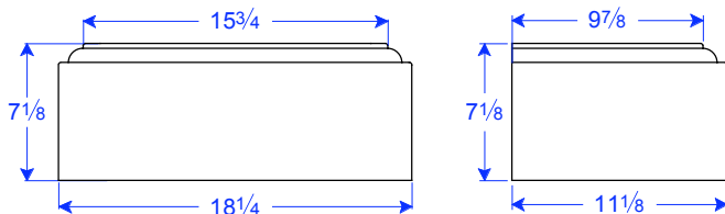
PL 18-15.75
