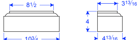
PL 18-8.5 x 4
