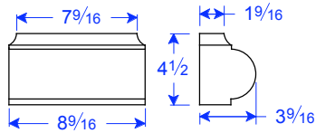
PL 01-7.56 x 4.5
