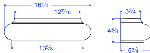
PL 01-12 x 4.5 DBN
