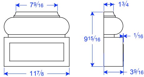
PL 01-7.56 x 9.6 DBN
