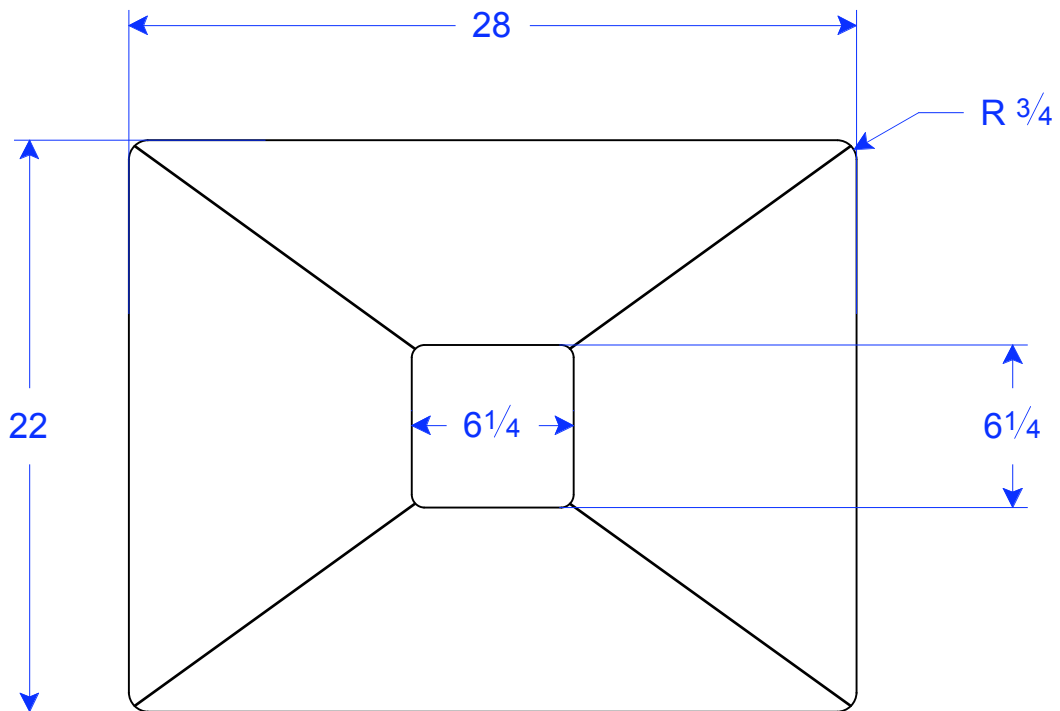
PC 01--22 P4.5 22"W x 28"L x 4 1/2"H(4+1/2)
