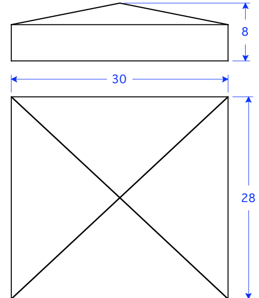
PC 13-28x30 P8 28"W x 30"L x 8"H
