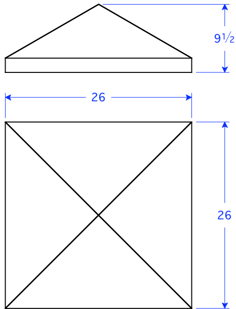
PC 13-26 P9.5 26"W x 26"L x 9 1/2"H
