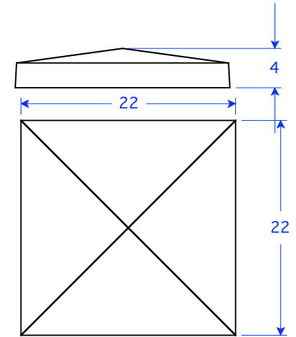
PC 13-22 P4 22"W X 22"L x 4"H.
