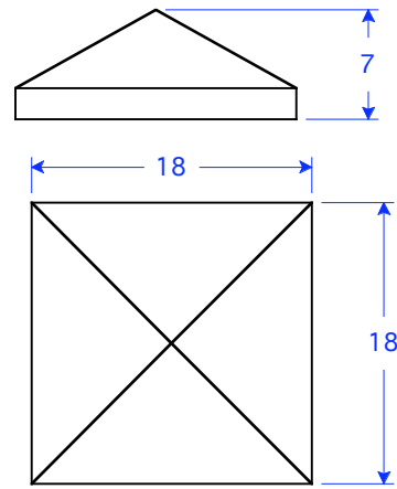
PC 13-18 P7 18"W x 18"L x 7"H
