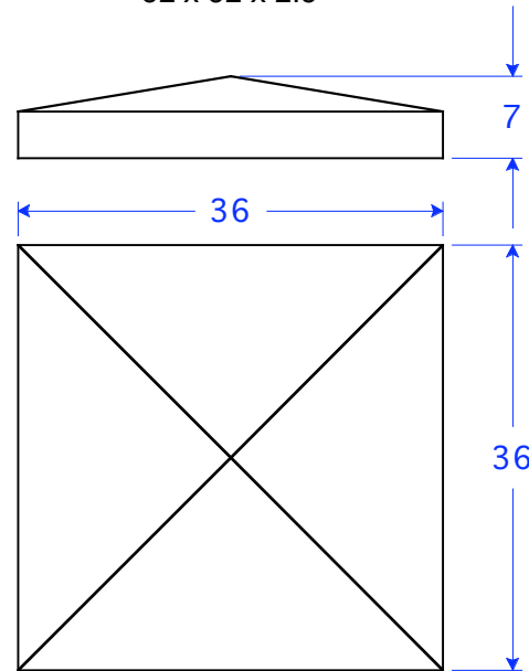
PC 13-36 P7 36"W x 36"L x 7"H
