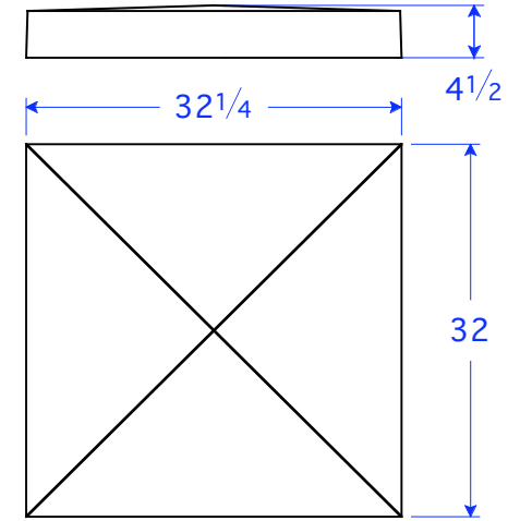
PC 13-32 P4.5 32"W x 32"L x 4 1/2"H
