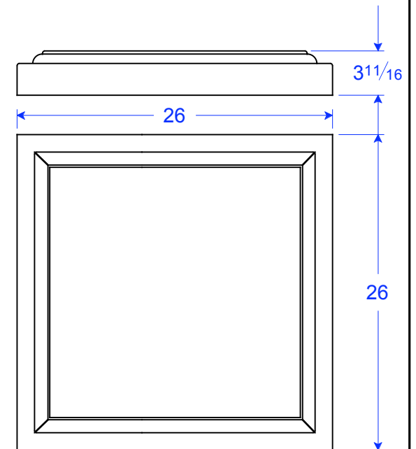
PC 18-26 F 26"W x 26"L x 3 11/16"
