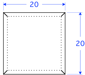
PC 36-20 BN F 17 1/2"W x 17 1/2"L x 3 1/4"H
