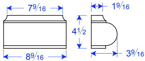
PL 01-7.56 x 4.5 8 9/16"W x 4 1/2"H x 3 9/16"D
