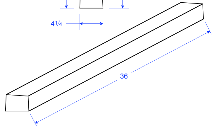
SM 02-04.25 STR 4 1/4"W x 36"L x 3"H
