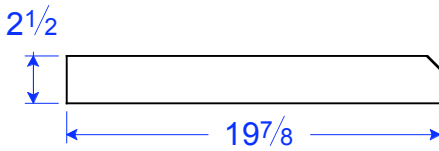
SM 23-19.875x2.5 STR 19.875"W x 24"L x 2 1/2"H
