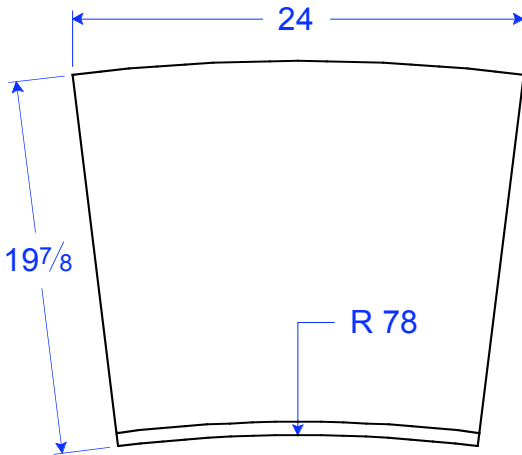
SM 23-19.875x2.5 STR R 78" 19.875"W x 24"L x 2 1/2"H
