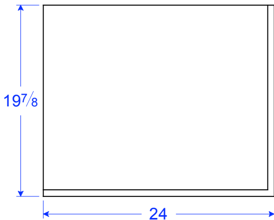
SM 23-19.875x2.5 CF 19.875"W x 24"L x 2 1/2"H
