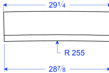
TM 20-5.5 R255" 8"H x 29 1/4"L x 5 1/2"T
