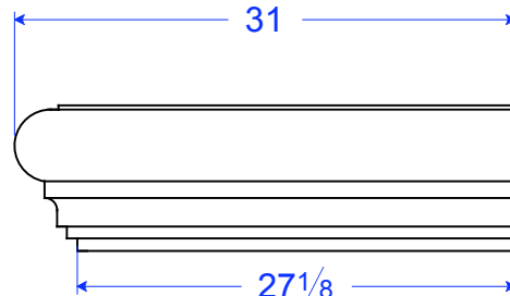
TM 21 LR 9"H x 31"L x 4 1/2"T
