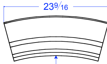
TM 21 STR R 37" 9"H x 23 9/16"L x 4 1/2"T
