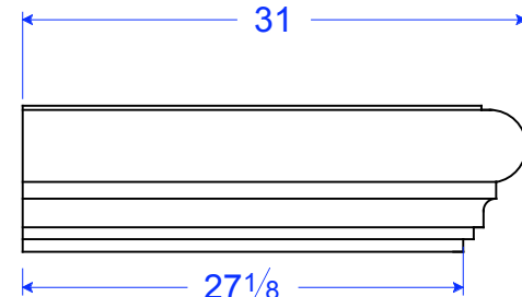
TM 21 RR 9"H x 31"L x 4 1/2"T
