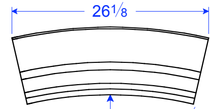
TM 21 STR R 50 3/16" 9"H x 26 1/8"L x 4 1/2"T
