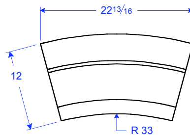
TM 22-12 STR R33 12"H x 22 13/16"L x 5"T
