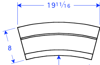
TM 22-8 STR R 30 1/2 8"H x 24-3/4"L x 4"T
