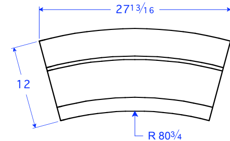
TM 22-12 STR R42 1/4 12"H x 27 13/16"L x 5"T
