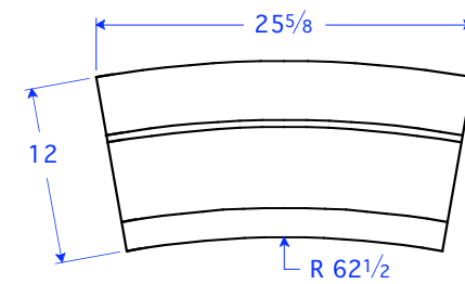
TM 22-12 STR R 62 1/2 12"H x 25 5/8"L x 5"T
