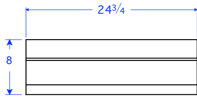
TM 22-8 STR 8"H x 24-3/4"L x 4"T
