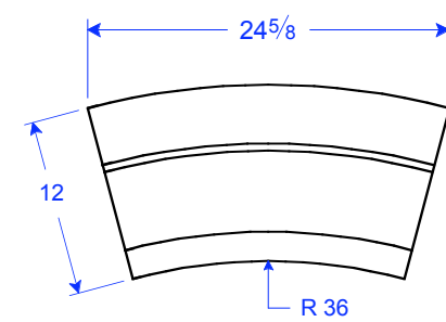
TM 22-12 STR R36 12"H x 24 5/8"L x 5"T
