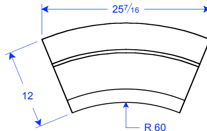
TM 22-12 STR R21 1/2 12"H x 25 7/16"L x 5"T
