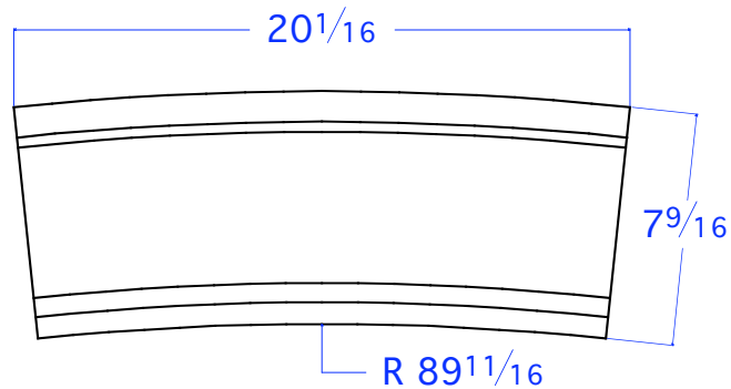
TM 23-8 STR R 89 11/16 7 9/16"W x 20 1/16+"L x 1 1/2"H
