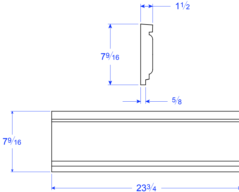
TM 23-8 STR 7 9/16"W x 23 3/4"L x 1 1/2"H
