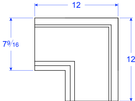
TM 23-8 CF 7 9/16"W x 12"Sq. x 1 1/2"H
