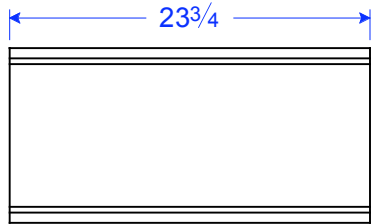
TM 24-12 STR 11 1/2"H x 23 3/4"L x 1 7/16"T
