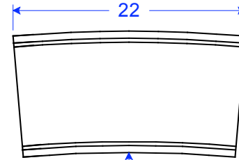
TM 24-12 STR R 119" 11 1/2"H x 22"L x 1 7/16"T
