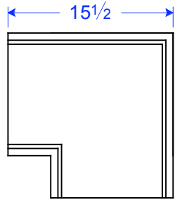
TM 24-12 CF 11 1/2"H x 15 1/2"SQ x 1 7/16"T
