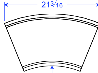
TM 24-12 STR R 16 1/2" 11 1/2"H x 21 3/16"L x 1 7/16"T
