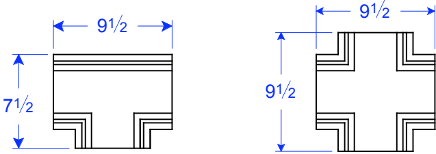
TM 24-5 T3 7 1/2"H x 9 1/2"L x 1 7/16"T
