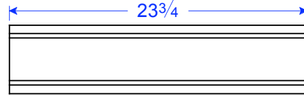
TM 24-5 STR 5 1/2"H x 23 3/4"L x 1 7/16"T
