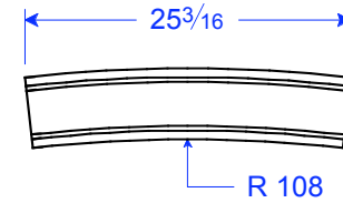
TM 24-5 STR R 108" 5 1/2"H x 25 3/16"L x 1 7/16"T
