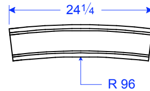
TM 24-5 STR R 96" 5 1/2"H x 24 1/4"L x 1 7/16"T
