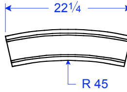
TM 24-5 STR R 45" 5 1/2"H x 22 1/4"L x 1 7/16"T
