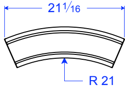
TM 24-5 STR R 21" 5 1/2"H x 21 1/16"L x 1 7/16"T
