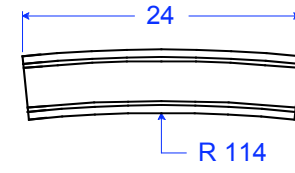
TM 24-5 STR R 114" 5 1/2"H x 24"L x 1 7/16"T
