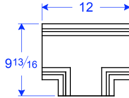
TM 24-8 T3 9 13/16"H x 12"L x 1 7/16"T
