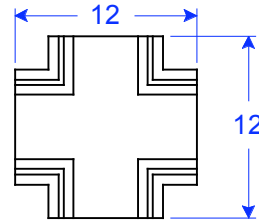
TM 24-8 T4 12"H x 12"L x 1 7/16"T
