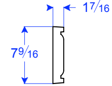
TM 24-8 STR 7 9/16"H x 23 3/4"L x 1 7/16"T
