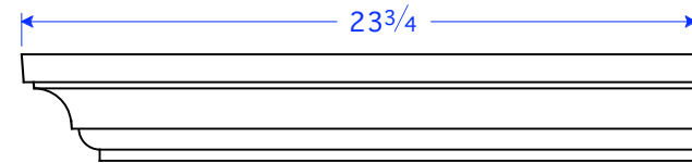
TM 26-6M LR 6"W x 23 3/4"L x 3 3/4"H
