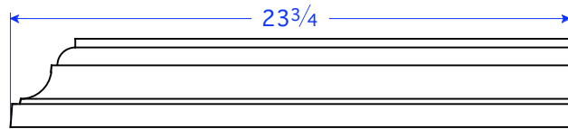
TM 26-6 LR 8 3/4"W x 23 3/4"L x 3 3/4"H
