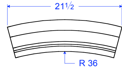
TM 30 STR R36 6"H x 21 1/2"L x 2 1/8"T
