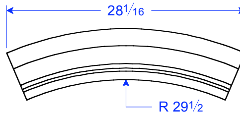
TM 30 STR R92.5 6"H x 28 1/16"L x 2 1/8"T
